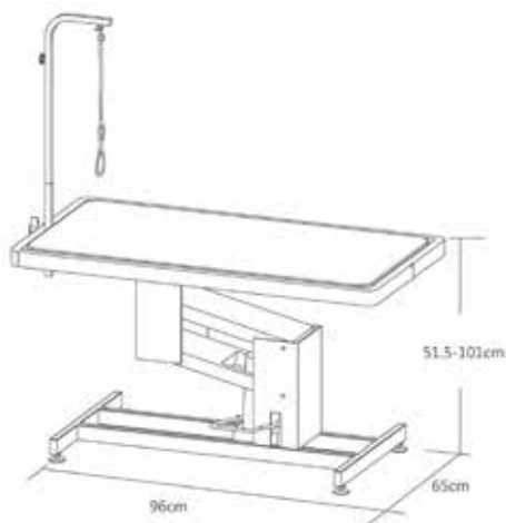
TOLE9834 tavolo idraulico 96x65xh51,5-101 cm
