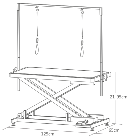
TOLE 9830 tavolo elettrico
