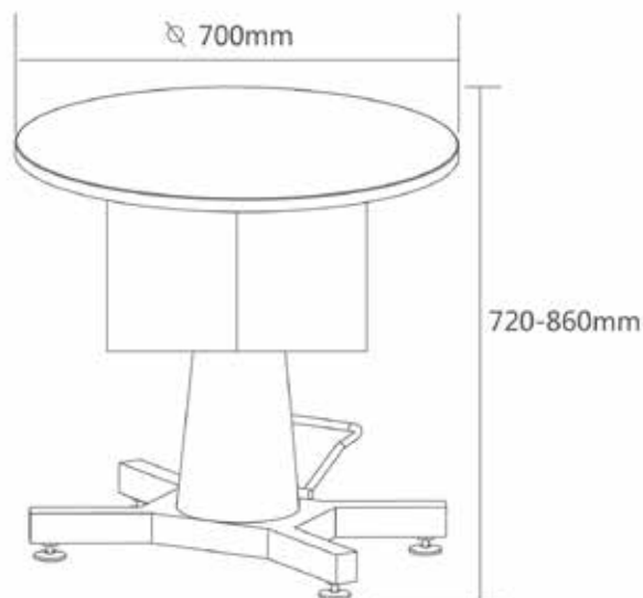
TOLE 9880 tavolo idraulico con cassetti
